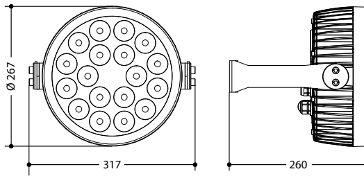
Disegno tecnico
