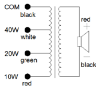
Schema elettrico
